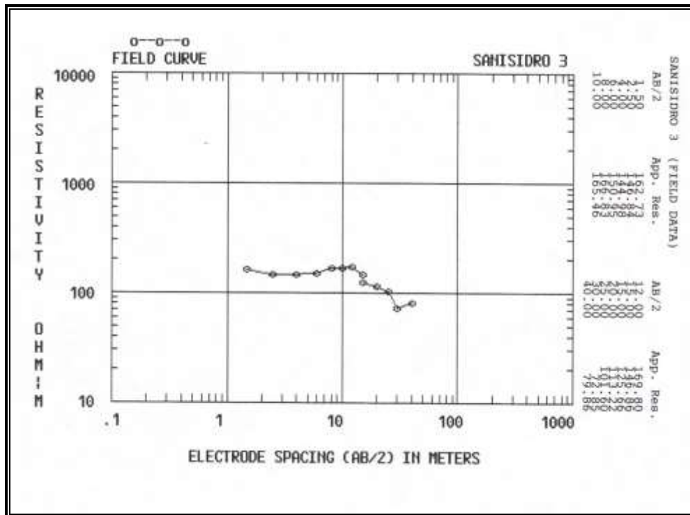
Figura D.5 Sondeo Eléctrico Vertical 3 – Resultados de Campo
