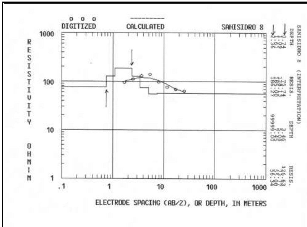
Figura D.16 Sondeo Eléctrico Vertical 8 – Interpretación
