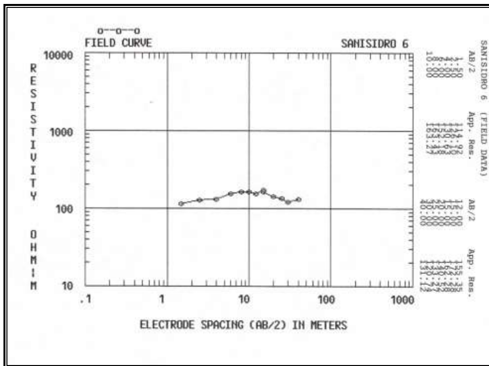
Figura D.11 Sondeo Eléctrico Vertical 6 – Resultados de Campo
