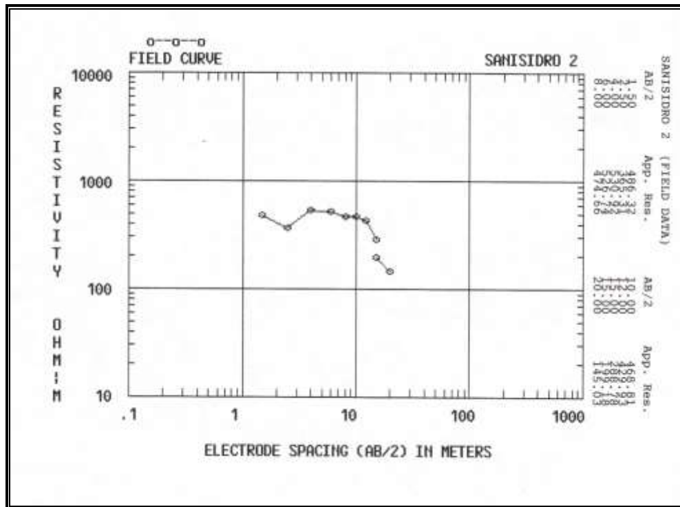
Figura D.3 Sondeo Eléctrico Vertical 2 – Resultados de Campo
