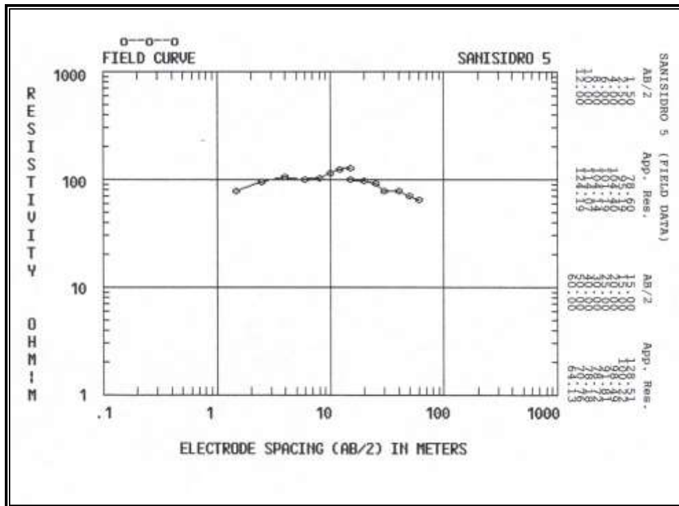
Figura D.9 Sondeo Eléctrico Vertical 5 – Resultados de Campo
