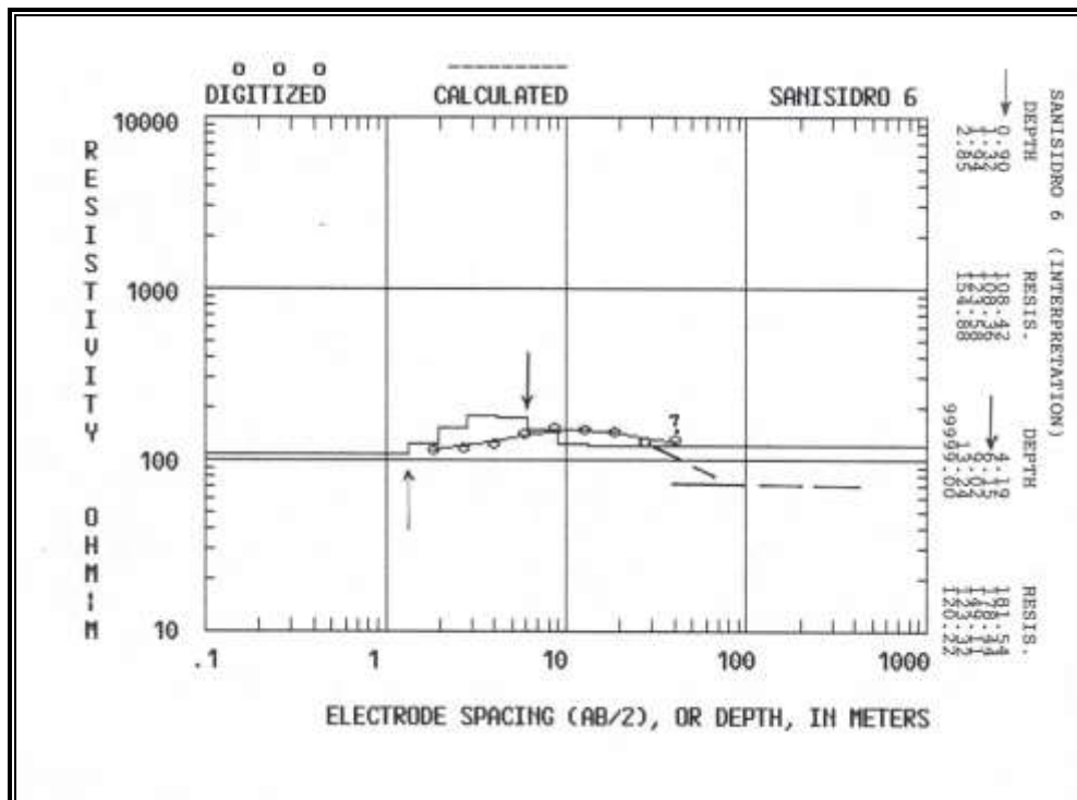
Figura D.12 Sondeo Eléctrico Vertical 6 – Interpretación
