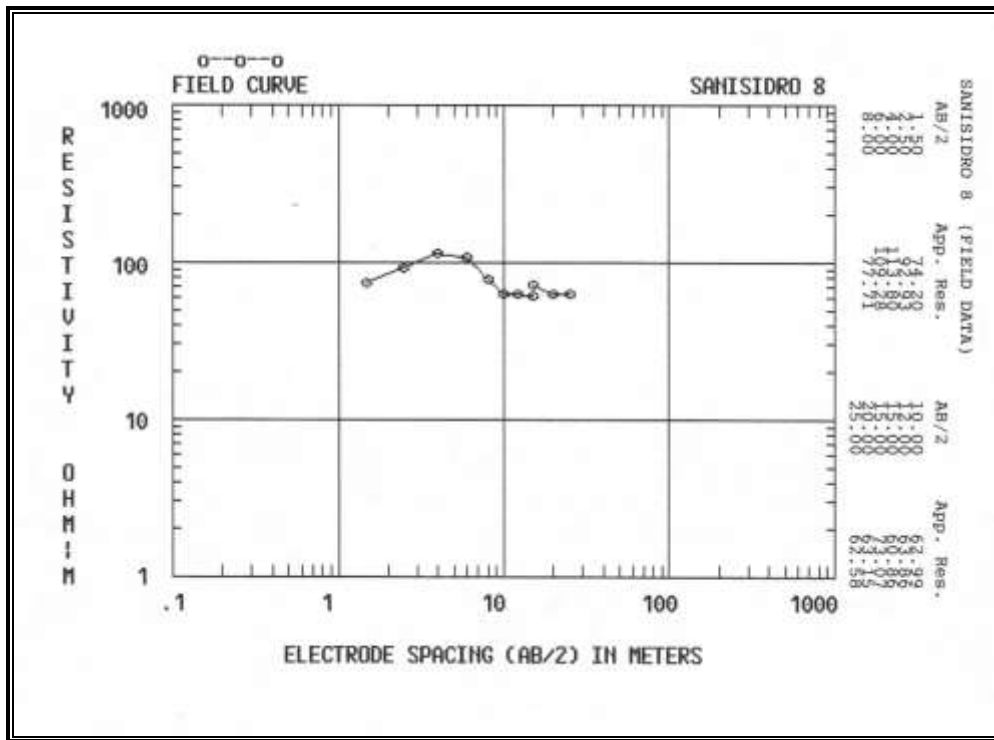
Figura D.15 Sondeo Eléctrico Vertical 8 – Resultados de Campo
