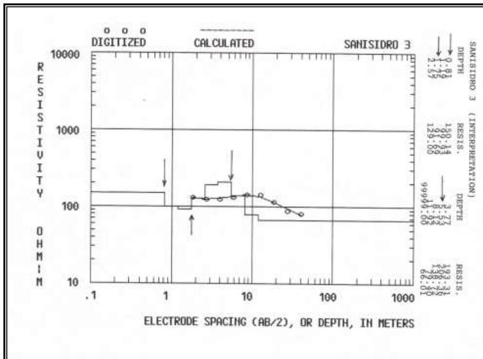
Figura D.6 Sondeo Eléctrico Vertical 3 – Interpretación
