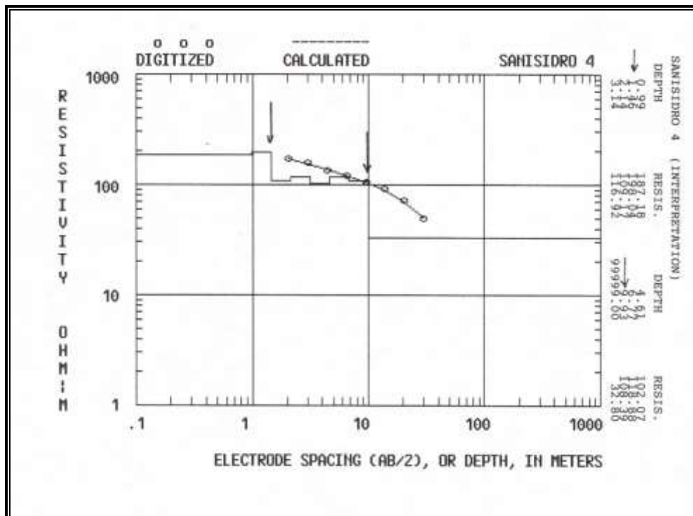
Figura D.8 Sondeo Eléctrico Vertical 4 – Interpretación
