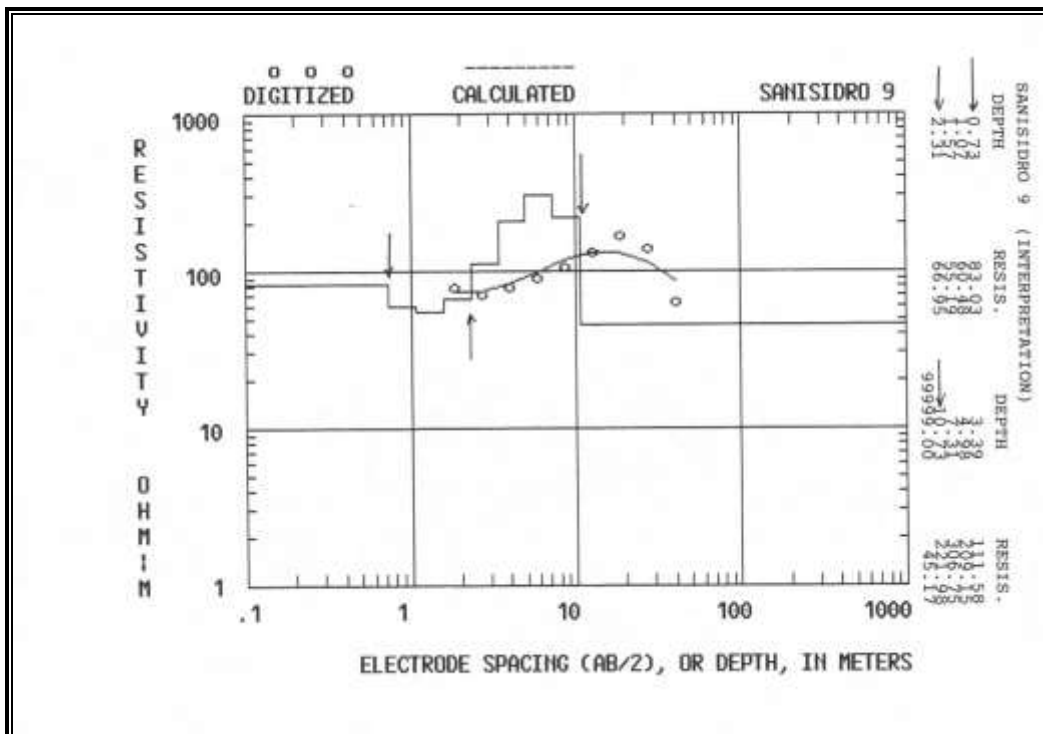
Figura D.18 Sondeo Eléctrico Vertical 9 – Interpretación
