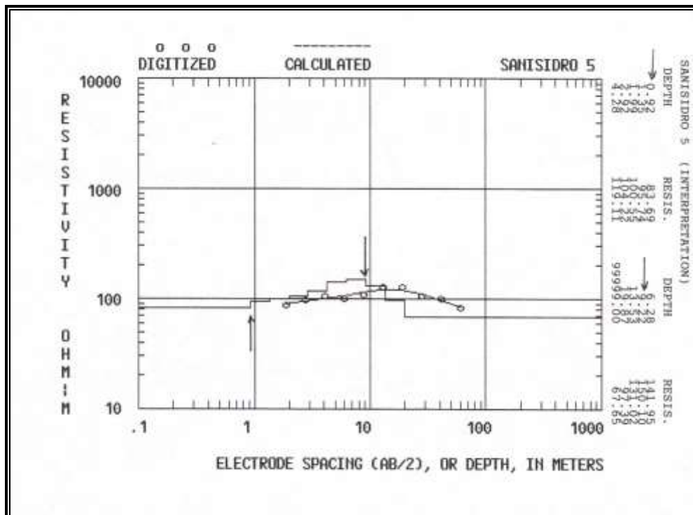
Figura D.10 Sondeo Eléctrico Vertical 5 – Interpretación
