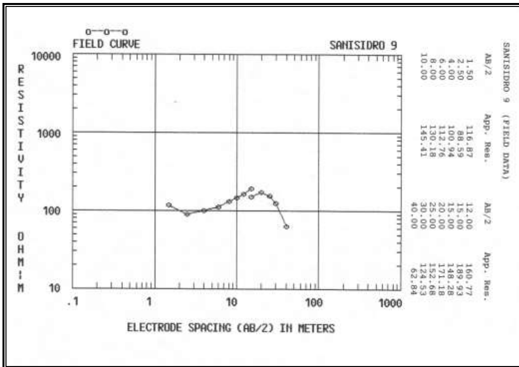
Figura D.17 Sondeo Eléctrico Vertical 9 – Resultados de Campo
