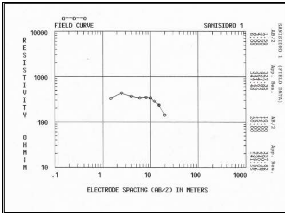
Figura D.1 Sondeo Eléctrico Vertical 1 – Resultados de Campo
