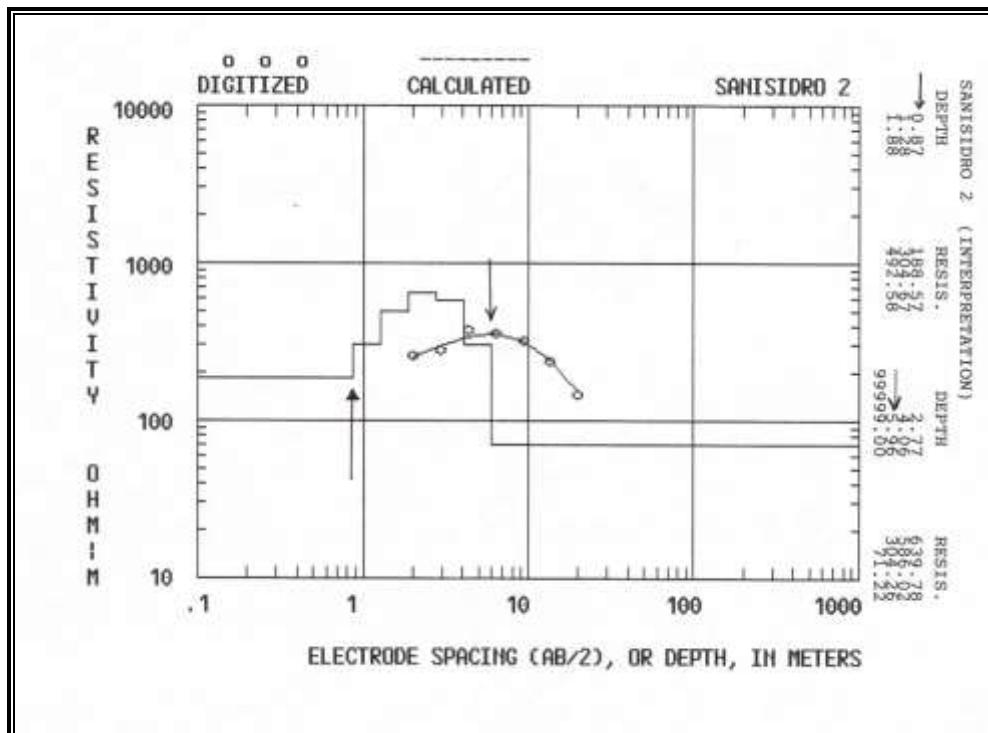
Figura D.4 Sondeo Eléctrico Vertical 2 – Interpretación
