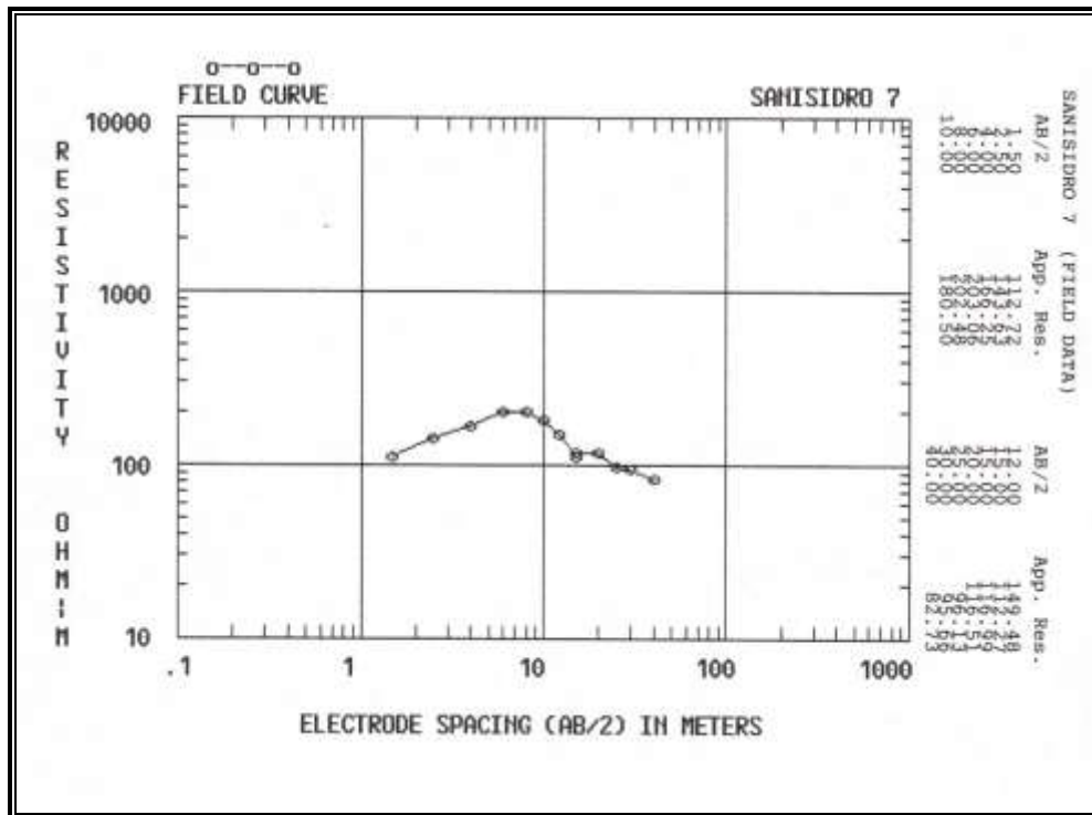
Figura D.13 Sondeo Eléctrico Vertical 7 – Resultados de Campo
