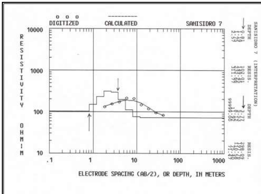
Figura D.14 Sondeo Eléctrico Vertical 7 – Interpretación
