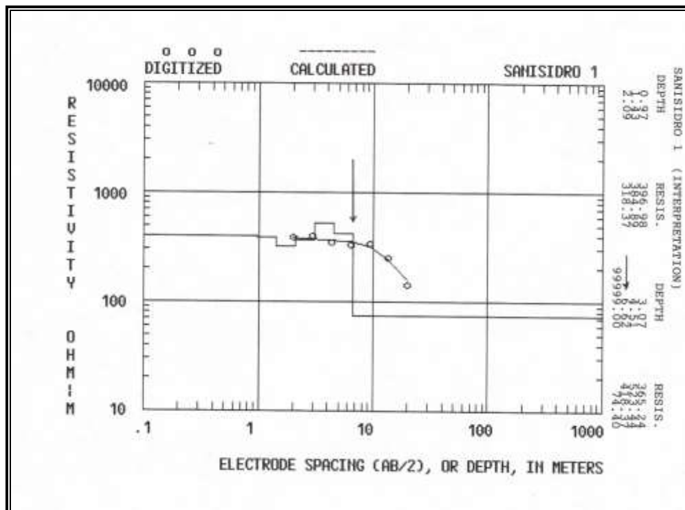
Figura D.2 Sondeo Eléctrico Vertical 1 – Interpretación
