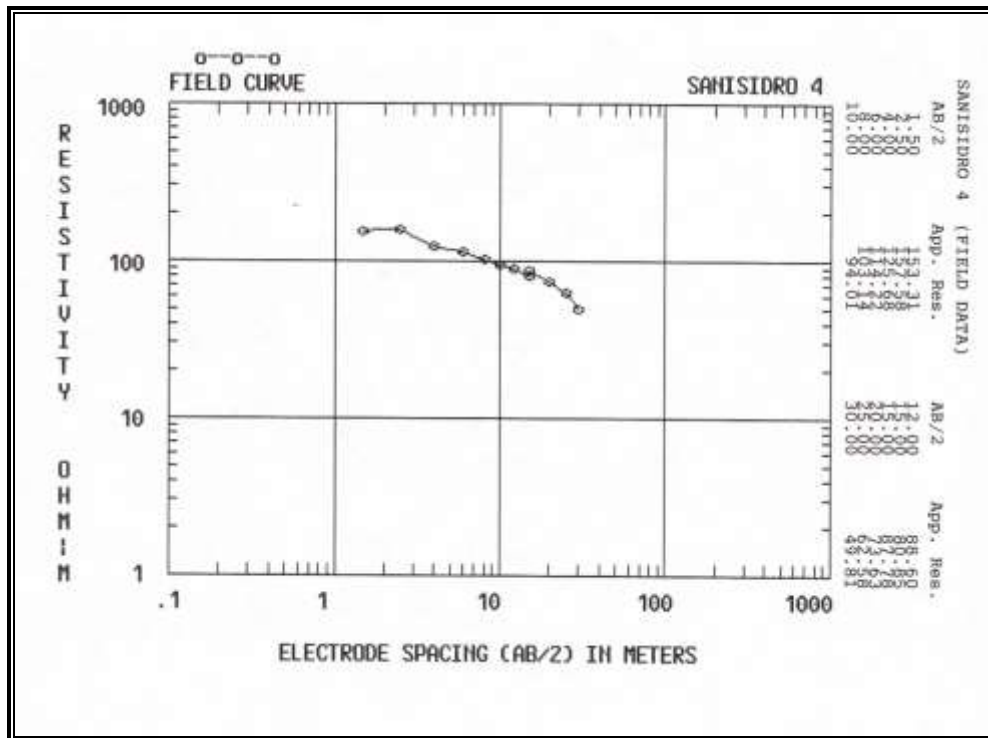
Figura D.7 Sondeo Eléctrico Vertical 4 – Resultados de Campo
