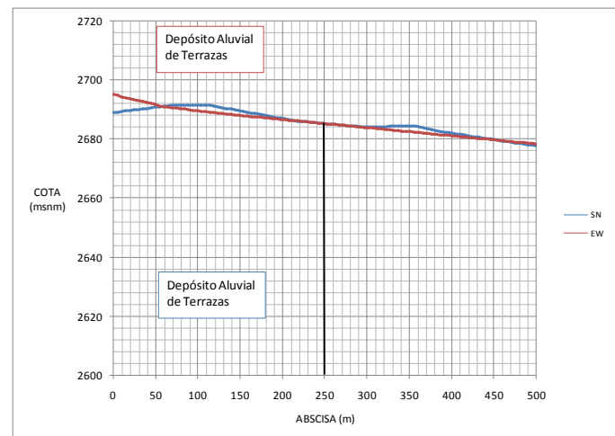
Figura 3.19. Perfil altimétrico Sur - Norte y Este - Oeste, estación "CMARI"
