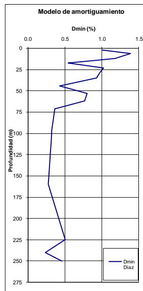
Figura 5.13. Modelo de respuesta 1D y resultados estación "CCITE"
