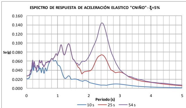
Figura 4.21. Espectro de respuesta de aceleraciones estación Centro de Estudios del Niño
