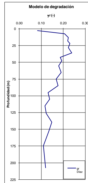
Figura 5.9. Modelo de respuesta 1D y resultados estación "CNINO"
