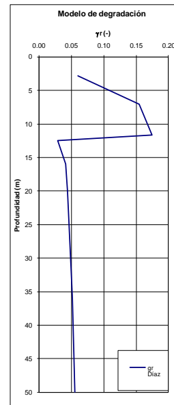
Figura 5.3. Modelo de respuesta 1D y resultados estación "CBANC"
