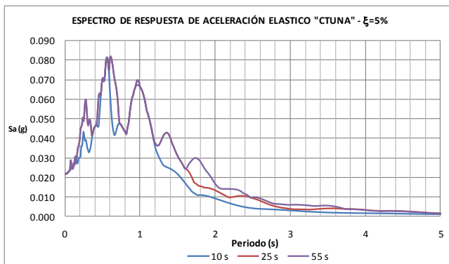
Figura 4.27. Espectro de respuesta de aceleraciones estación Tunal
