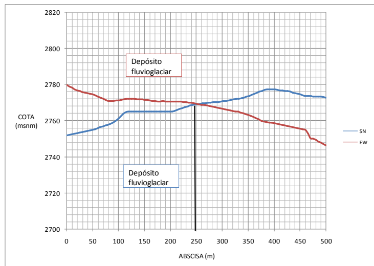
Figura 3.23. Perfil altimétrico Sur – Norte y Este – Oeste, estación “CVITE”
