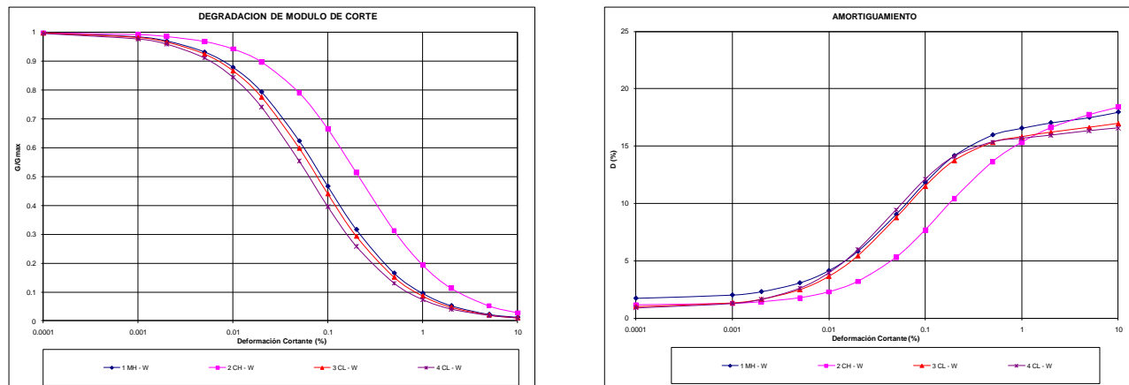
Figura 6.4. Curvas dinámicas segmento occidental – modelo norte
