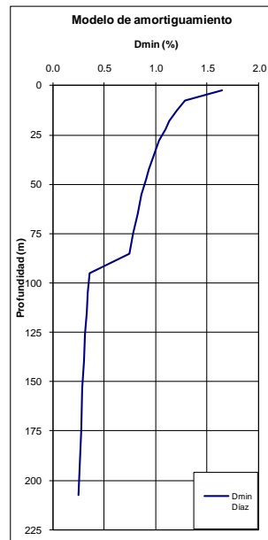
Figura 5.9. Modelo de respuesta 1D y resultados estación "CNINO"
