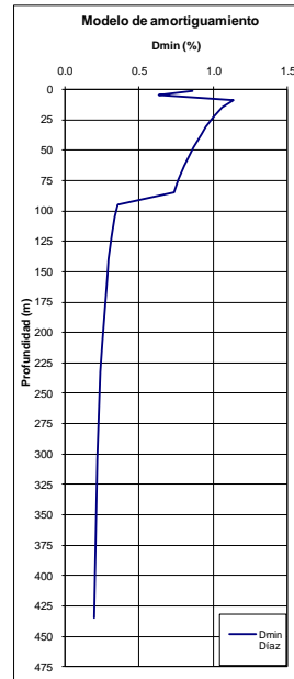
Figura 5.11. Modelo de respuesta 1D y resultados estación "CFLOD"
