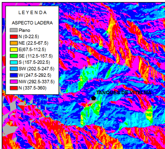
Figura 3.22. Aspecto de ladera “CVITE”
