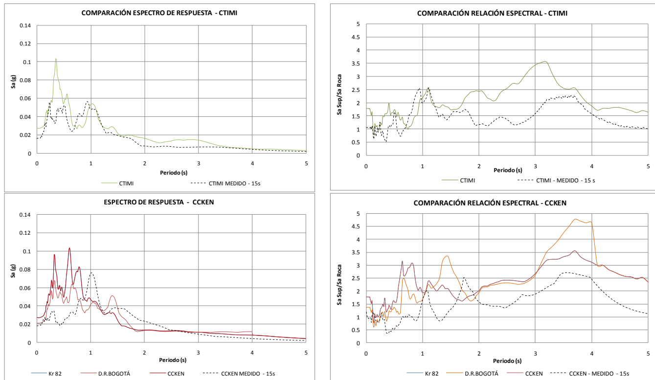
Figura 6.22. Comparación respuesta medidas y modeladas – modelo sur
