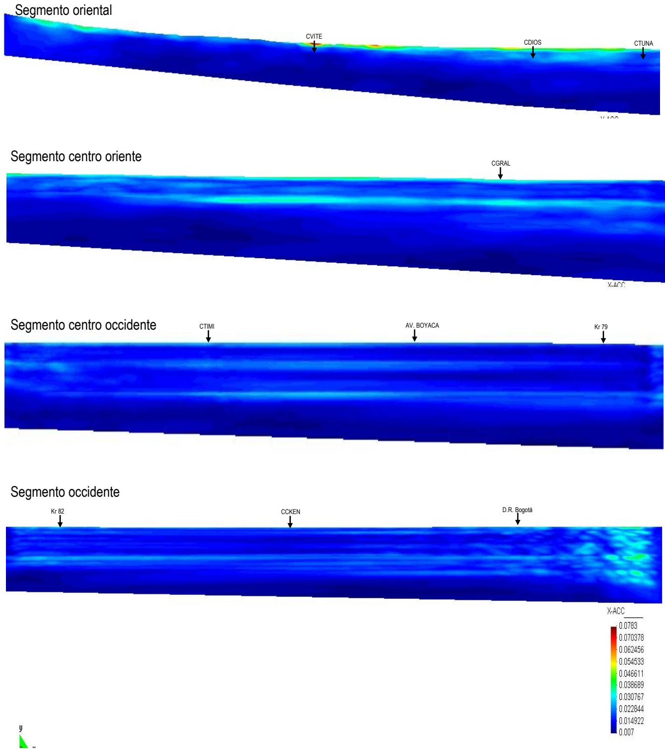
Figura 6.20. Aceleraciones máximas – modelo sur
