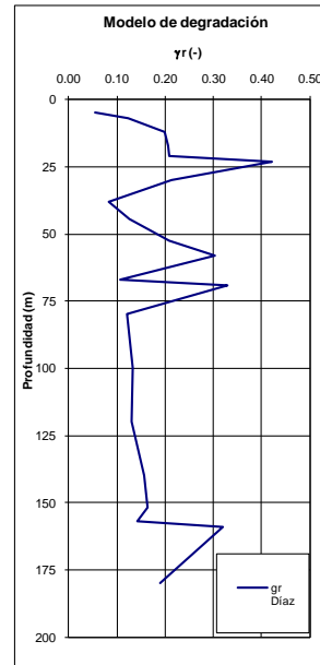
Figura 5.6. Modelo de respuesta 1D y resultados estación "CBOG1"
