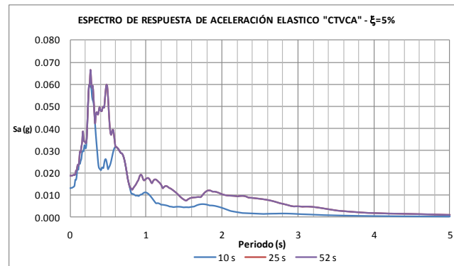
Figura 4.8. Espectro de respuesta de aceleraciones estación TVCABLE
