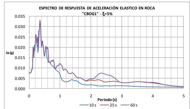
Figura 4.18. Espectro de respuesta de aceleraciones estación Ingeominas - Roca
