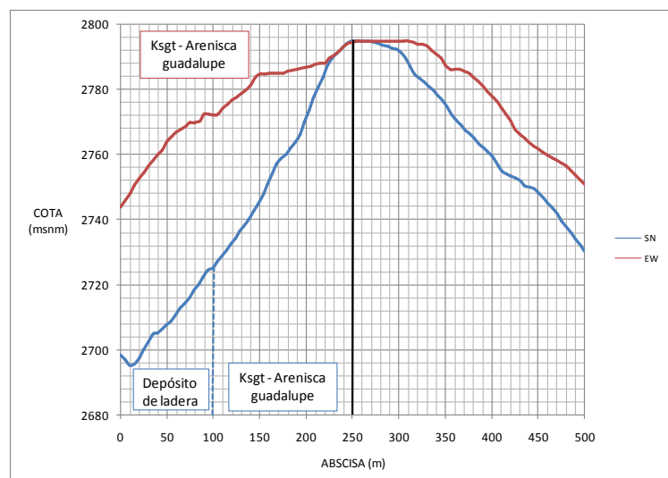
Figura 3.21. Perfil altimétrico Sur – Norte y Este – Oeste, estación “CSMOR”
