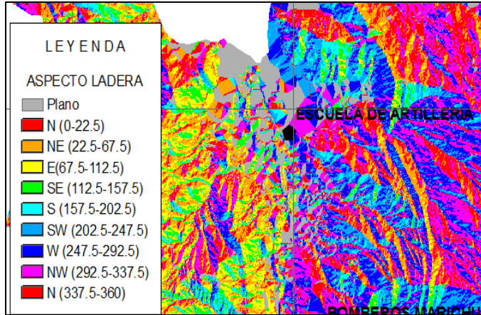
Figura 3.16. Aspecto de ladera "CARTI"
