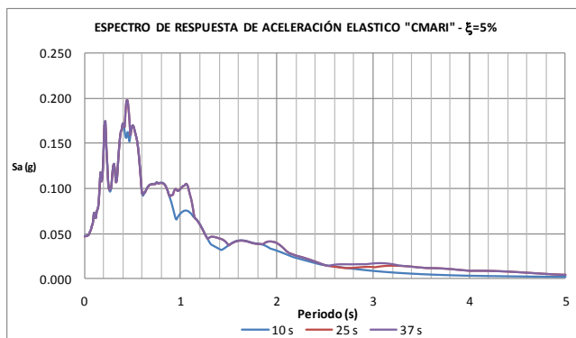
Figura 4.9. Espectro de respuesta de aceleraciones estación Bomberos Marichuela.
