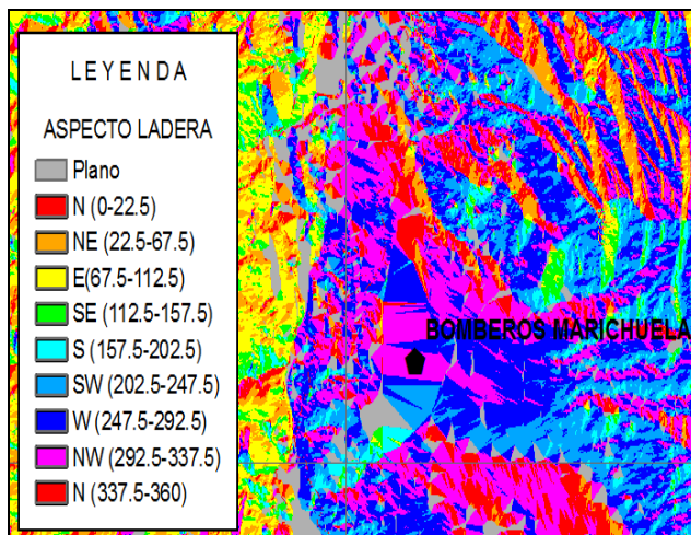
Figura 3.18. Aspecto de ladera "CMARI"
