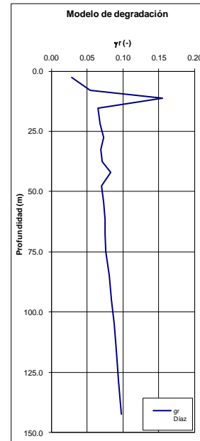
Figura 5.17. Modelo de respuesta 1D y resultados estación "CTIMI"
