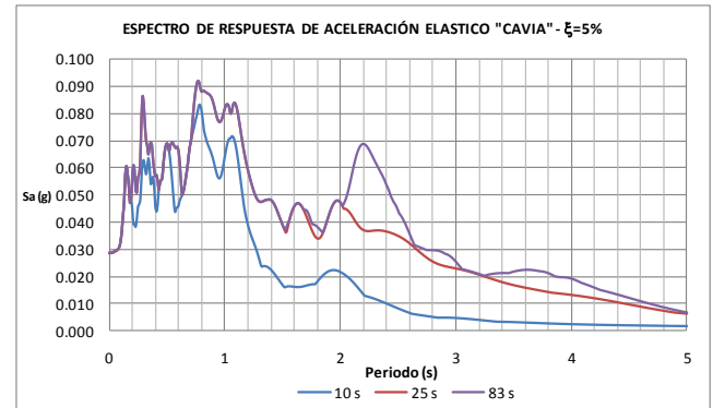
Figura 4.22. Espectro de respuesta de aceleraciones estación Avianca
