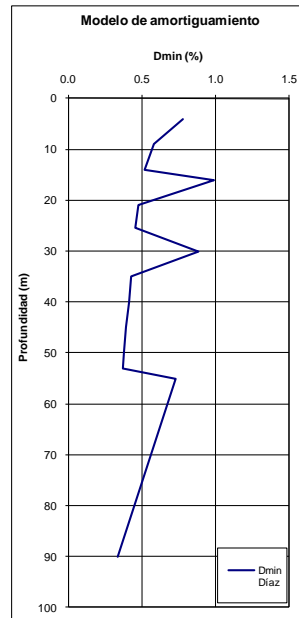
Figura 5.19. Modelo de respuesta 1D y resultados estación "CGRAL"
