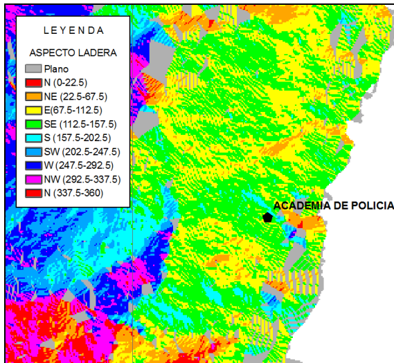
Figura 3.4. Aspecto de ladera “CPSUB”
