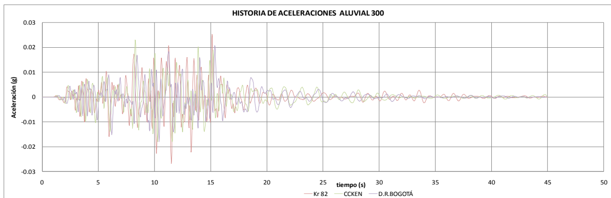
Figura 6.18. Historia de aceleraciones – modelo sur
