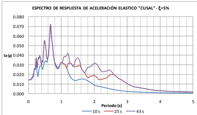
Figura 4.11. Espectro de respuesta de aceleraciones estación Universidad de la Salle.
