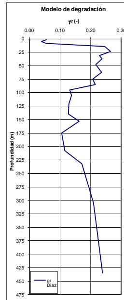
Figura 5.11. Modelo de respuesta 1D y resultados estación "CFLOD"
