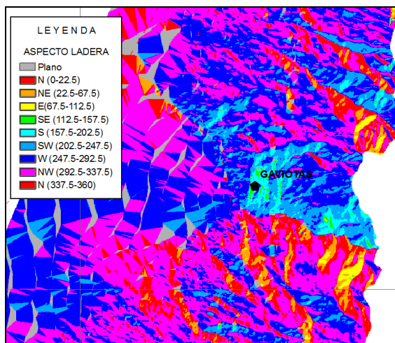
Figura 3.24. Aspecto de ladera “CBOG2”
