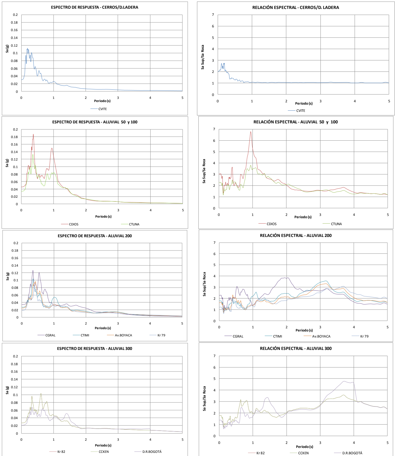
Figura 6.19. Espectros y relaciones espectrales – modelo sur
