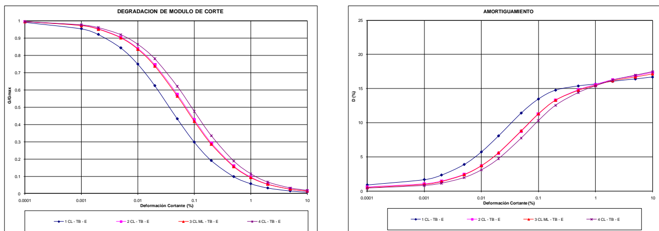
Figura 6.14. Curvas dinámicas terraza baja segmento oriental – modelo sur
