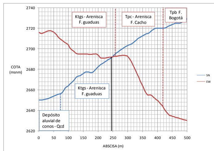
Figura 3.25. Perfil altimétrico Sur – Norte y Este – Oeste, estación “CBOG2”
