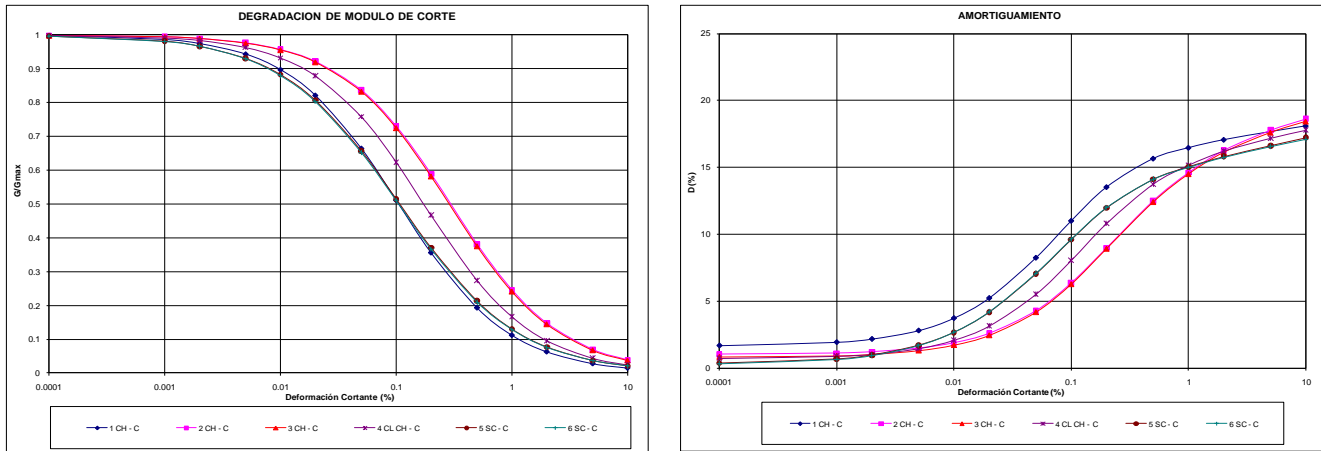
Figura 6.5. Curvas dinámicas segmento central – modelo norte
