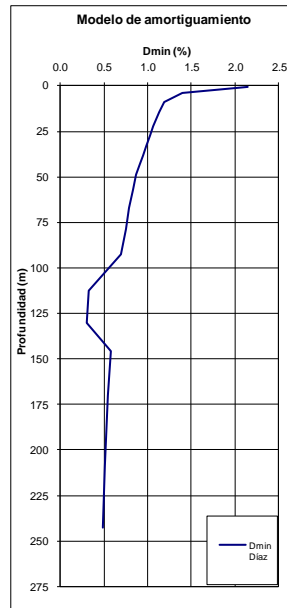
Figura 5.7. Modelo de respuesta 1D y resultados estación "CCORP"
