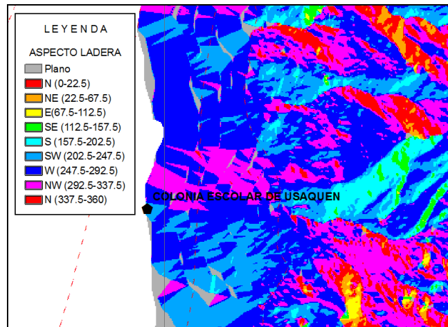
Figura 3.6. Aspecto de ladera “CUSAQ”
