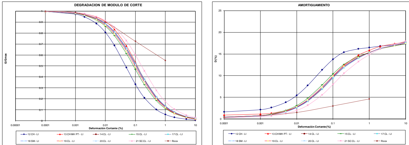
Figura 6.17. Curvas dinámicas segmento occidental llanura inundación – modelo sur
