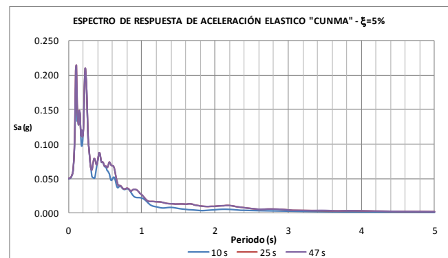
Figura 4.10. Espectro de respuesta de aceleraciones estación Universidad Manuela Beltrán
