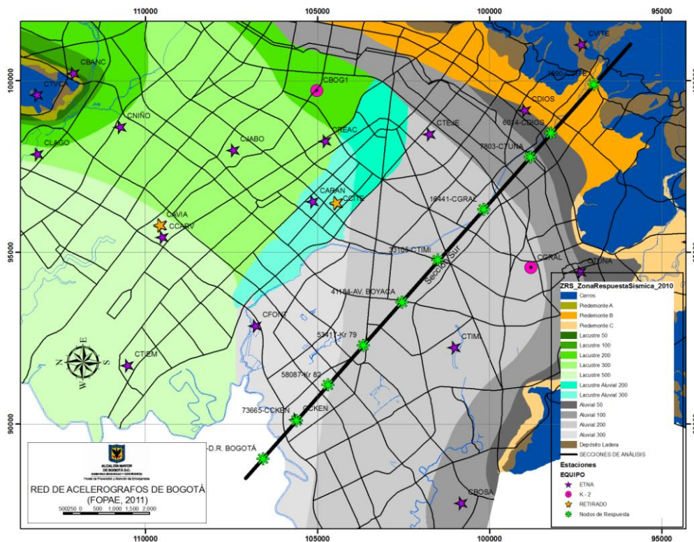
Figura 6.12. Localización del modelo bidimensional al sur
