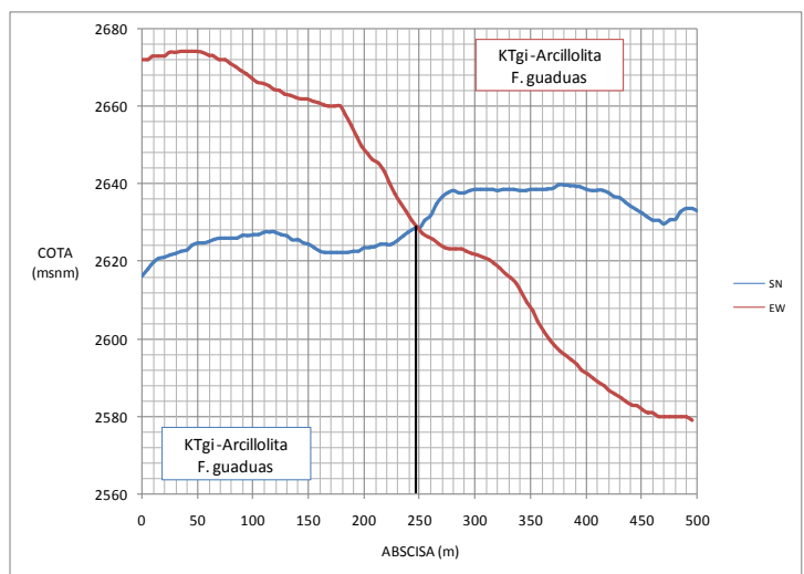
Figura 3.10. Perfil altimétrico Sur – Norte y Este – Oeste, estación “CTVCA”
