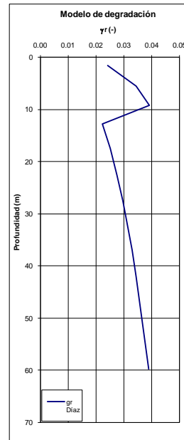
Figura 5.15. Modelo de respuesta 1D y resultados estación "CTUNA"
