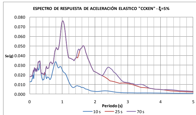
Figura 4.33. Espectro de respuesta de aceleraciones estación Col. Kennedy
