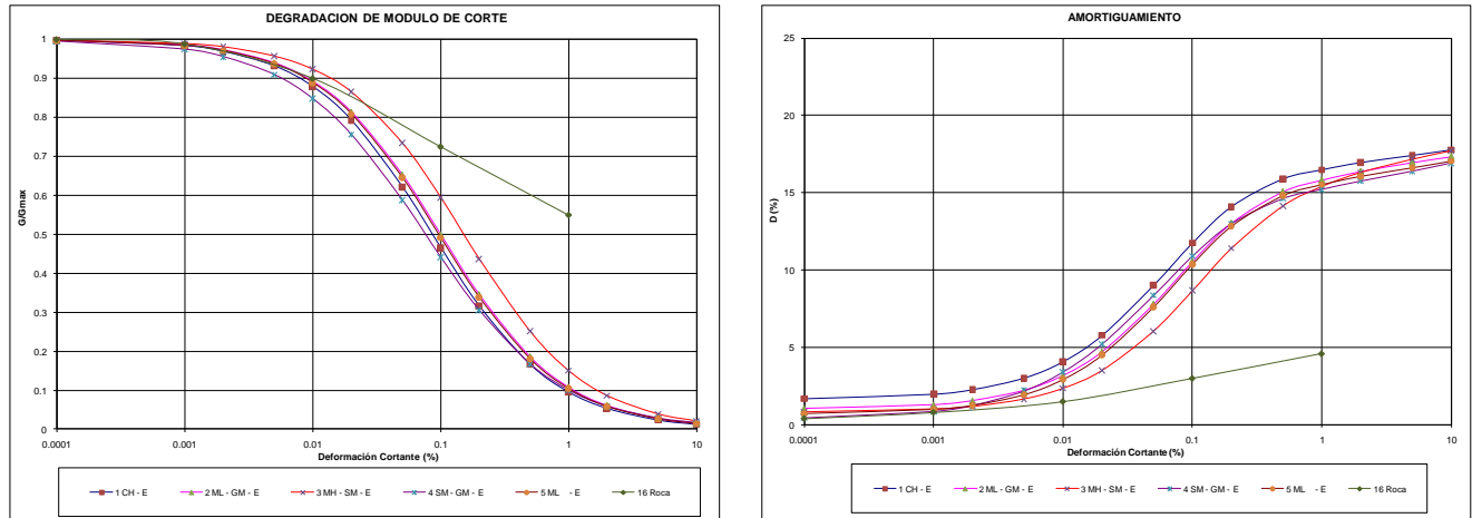
Figura 6.6. Curvas dinámicas segmento oriental – modelo norte
