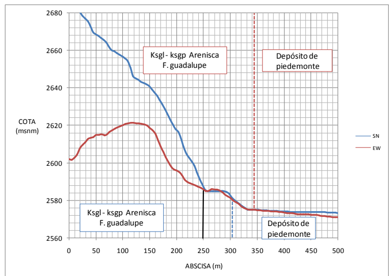
Figura 3.8. Perfil altimétrico Sur – Norte y Este – Oeste, estación “CESCA”
