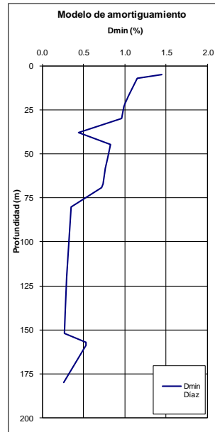
Figura 5.6. Modelo de respuesta 1D y resultados estación "CBOG1"
