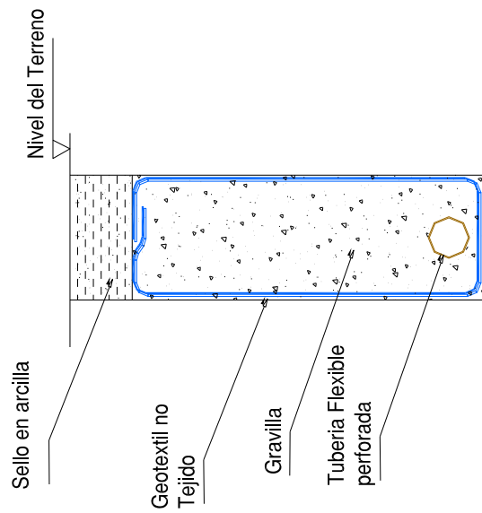
Alternativa de Subdrén con Gravilla
