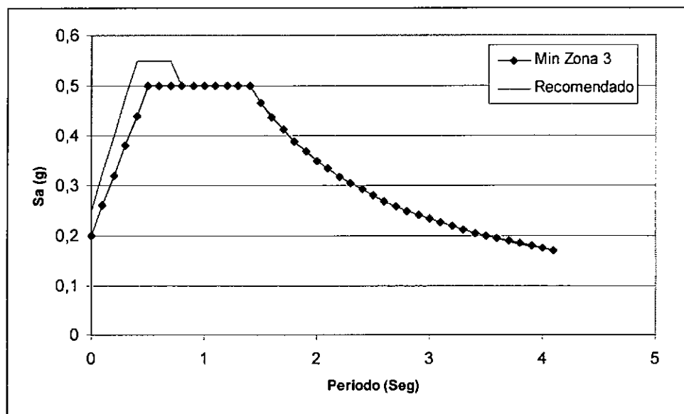
Figura 2. Espectro de diseño recomendado proyectos Urbanización Andalucía y Balcones de San Carlos
